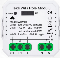
Tekli Anahtar Modülü
