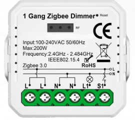
Dimmer Anahtar Modülü
